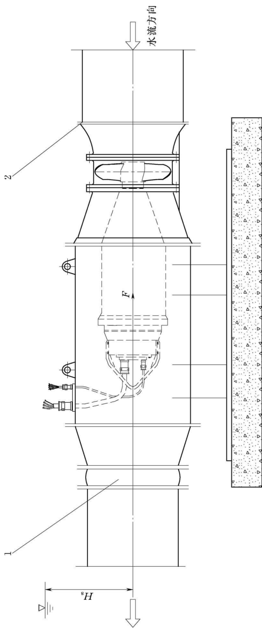
c) 贯流式潜水泵管道式安装
