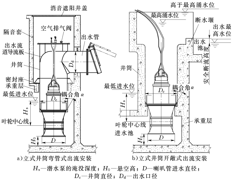
图 3.4.3 立式潜水泵井筒式典型安装
