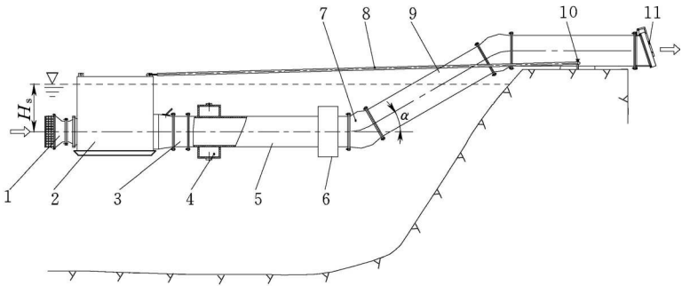
1—潜水泵；2—潜水泵浮箱；3、7—挠性接头；4—浮力调节阀；5—浮力出水管；6—出水管浮箱；8—缆绳；9—出水管；10—栓桩；11—拍门
