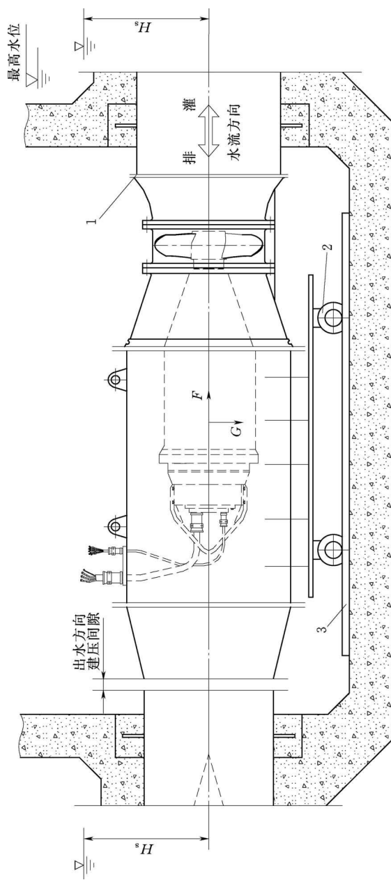
b) 贯流式潜水泵排灌结合双向承插式安装 1—止水密封圈；2—车轮；3—导轨； H_s —潜水泵的淹没深度 图 3.4.2 贯流式潜水泵安装 (二)
